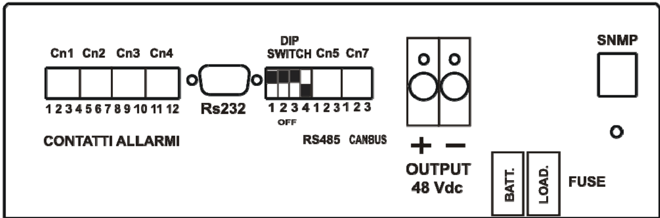
PANNELLO CONNESSIONI
